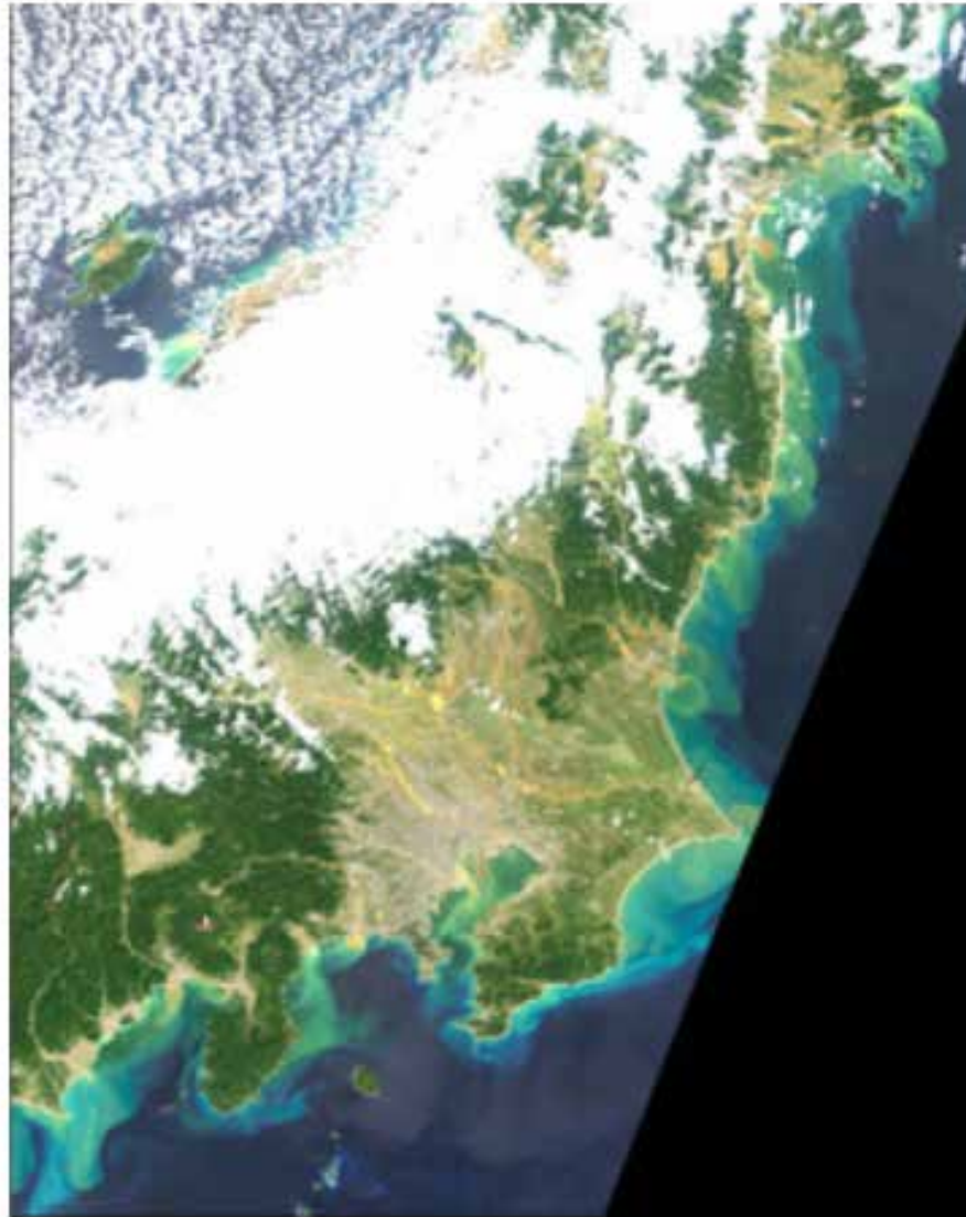
気候変動観測衛星「しきさい」が13日午前10時50分ごろに撮影した日本（JAXA提供）
